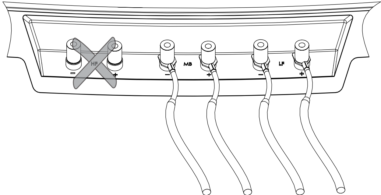
Bornes arrière
